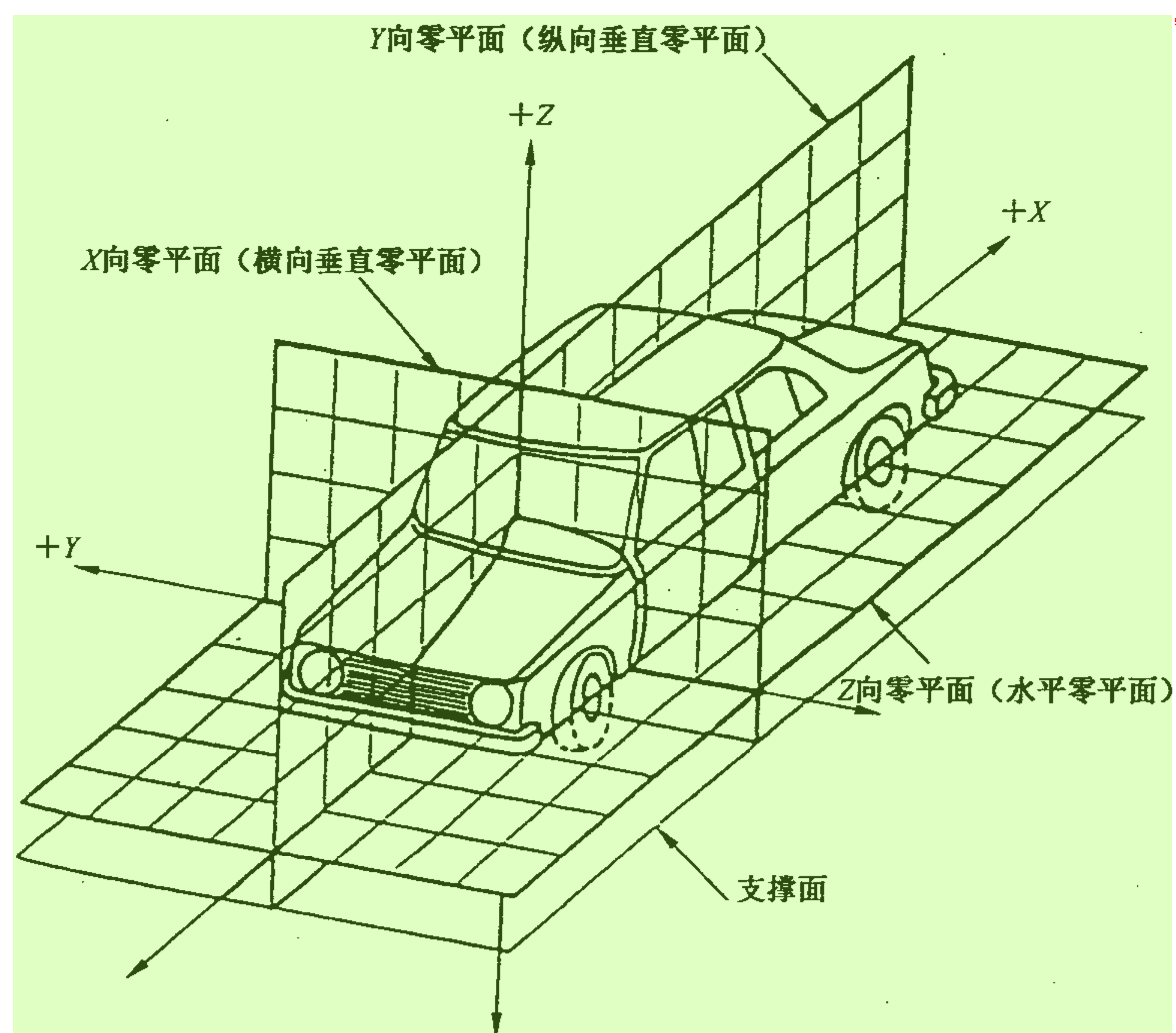
图 A.3 三维坐标系 5
