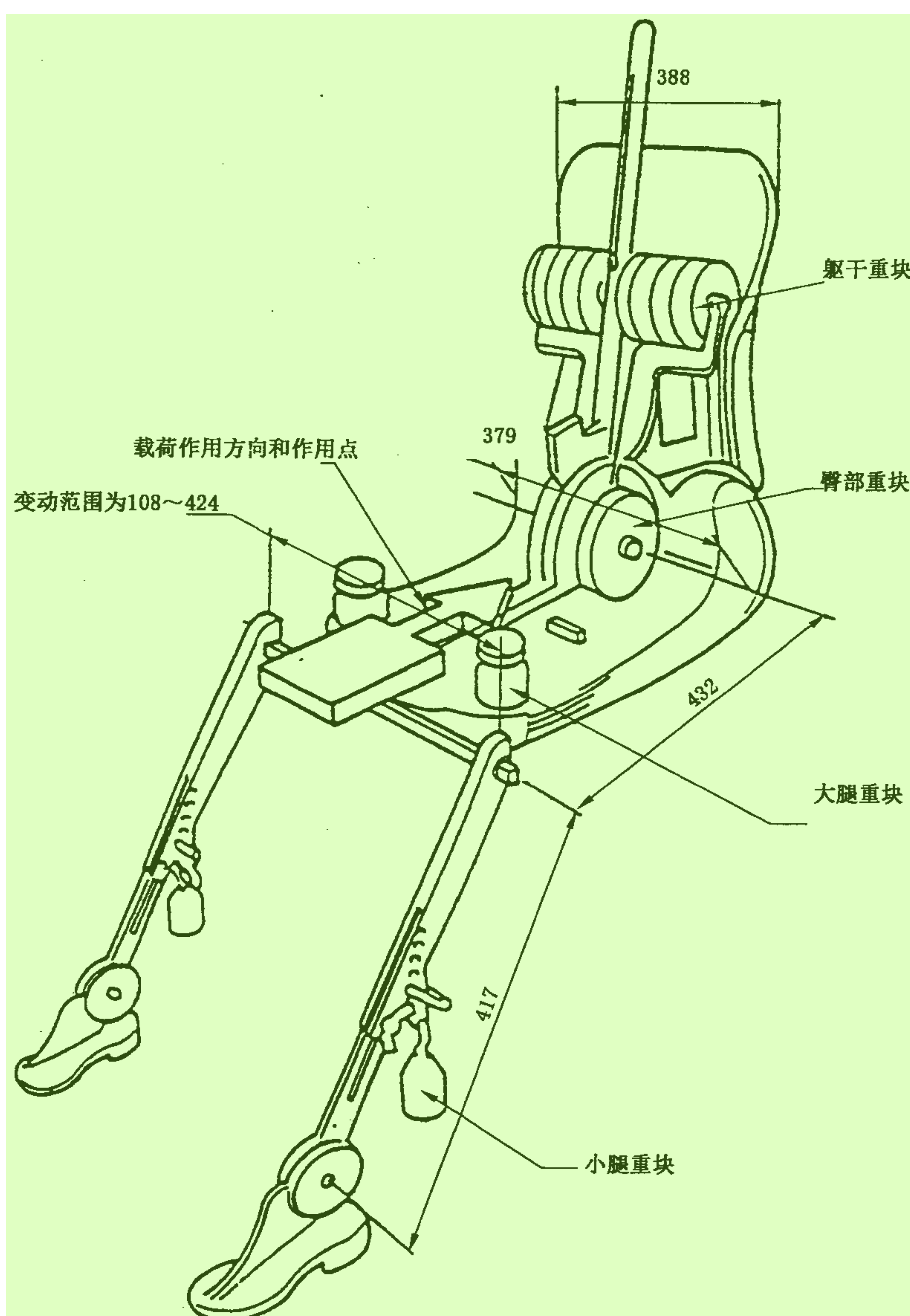
图 A.2 3-D H 装置构件尺寸和负荷分布 11
