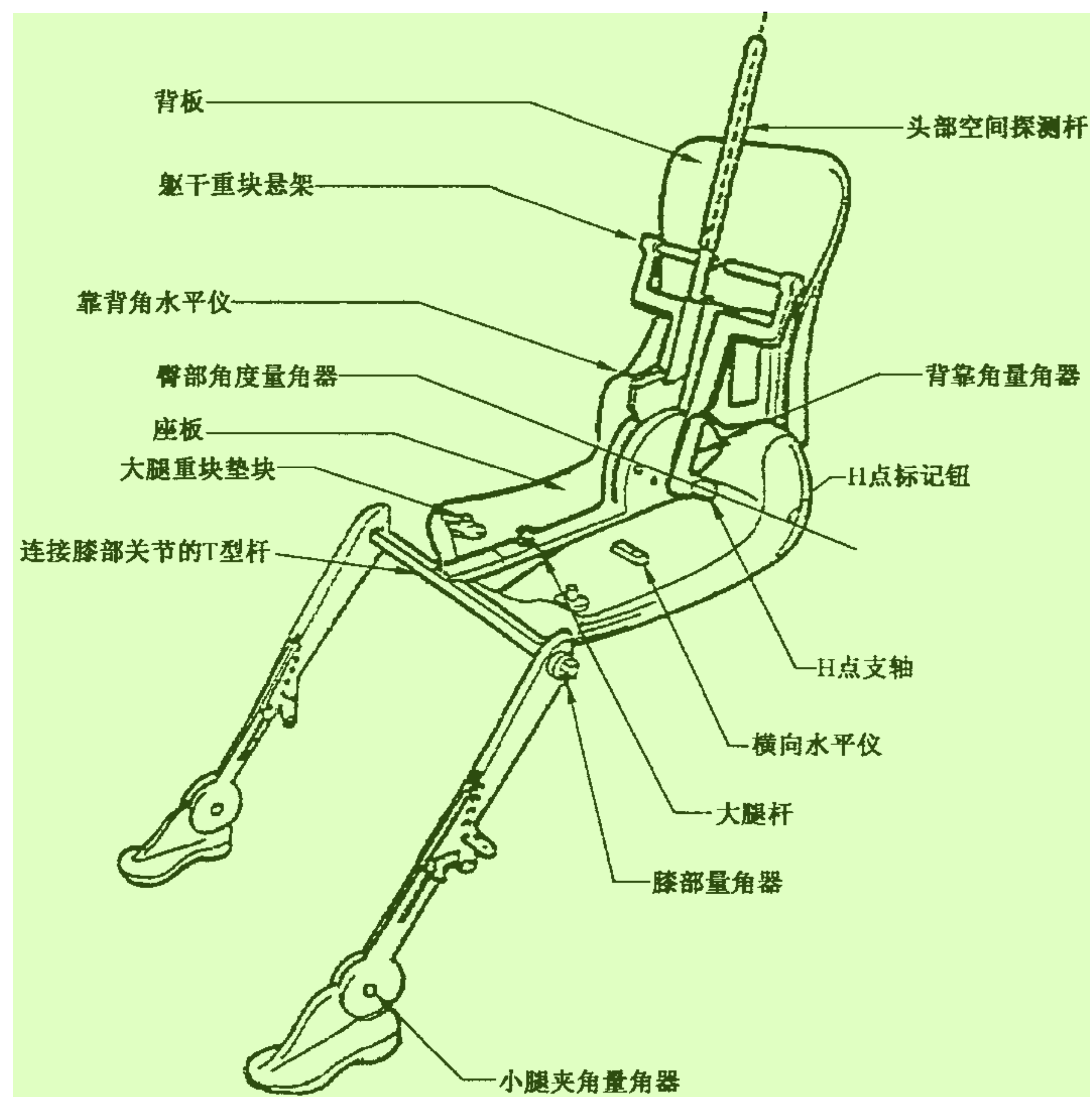
图 A.1 3-D H 装置构件名称
