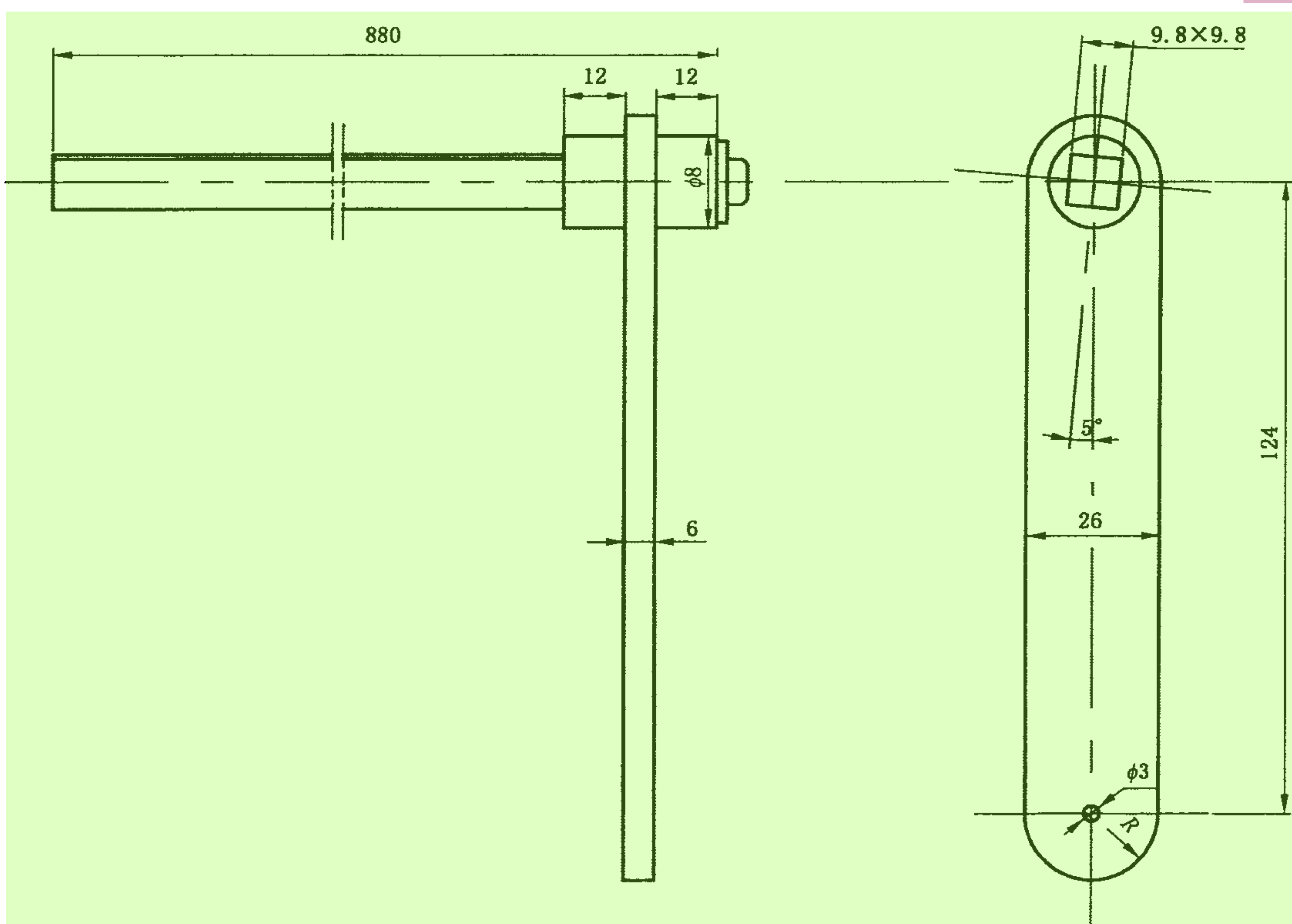
图 C.1 骨盆角度量规 8
